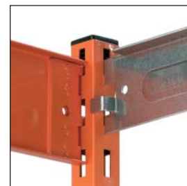
Gesamtstabilisierung durch Längsverbände und Auflagetraversen.
