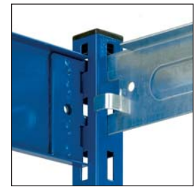
Gesamtstabilisierung durch Längsverbände und Auflagetraversen.
