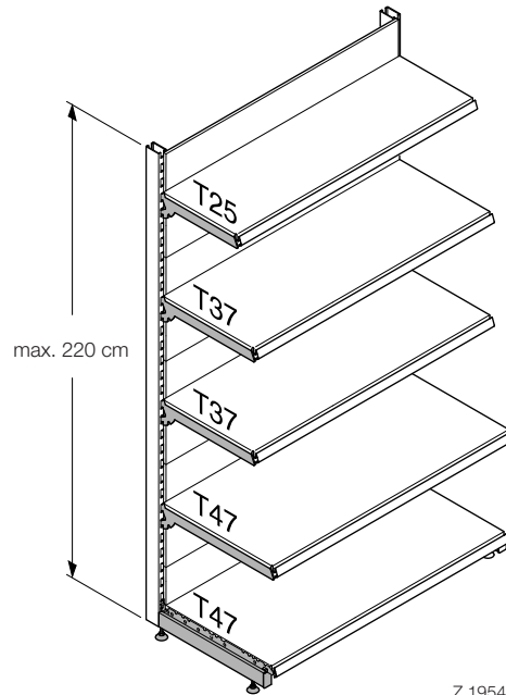
Abb. 1 Wandregalständer mit einer mittleren Tiefe T von 37 und einem Fußteilboden T 47.
